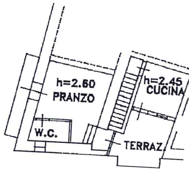
PIANTA P.SECONDO
